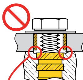
Deformação do plástico
