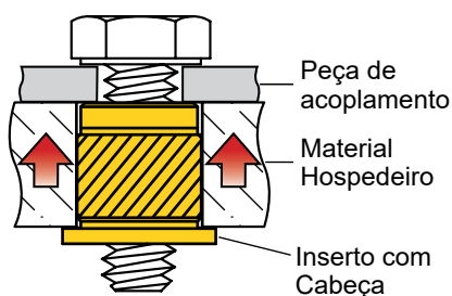
Configuração Instalação Reversa
