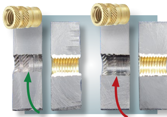
Figura 1: Fluxo de plástico adequado
